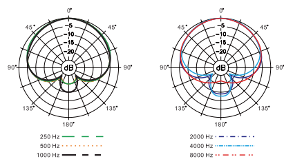
D103 频率响应图
